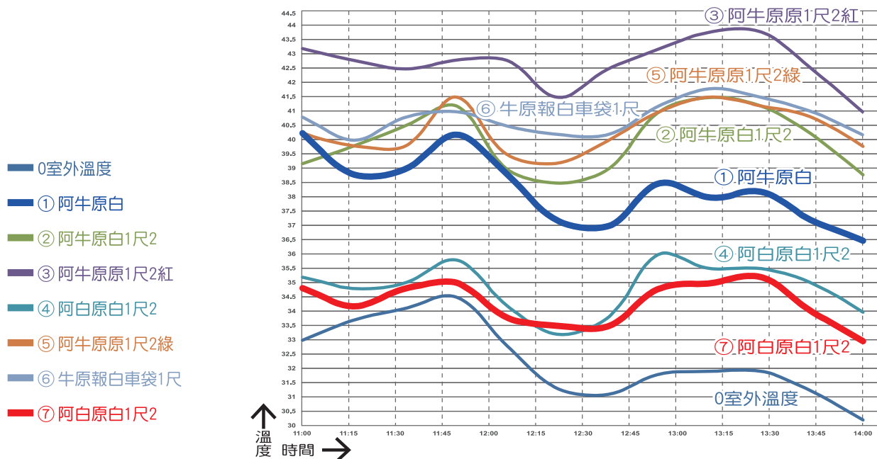
阿不倒袋內溫度田間實測曲線圖
